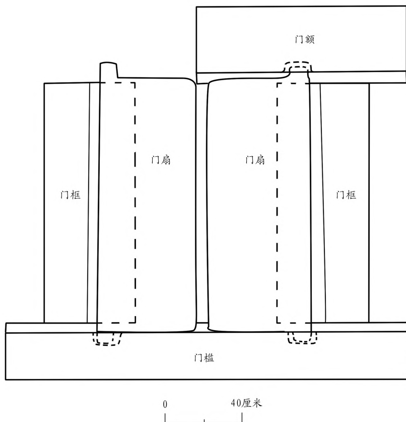
图四// M2石门立面图
