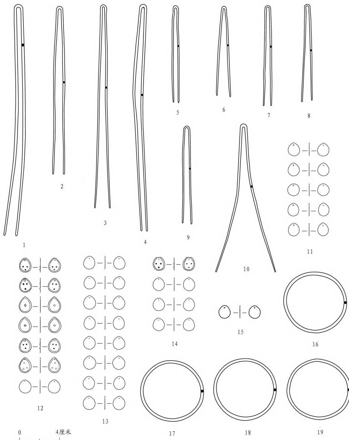
图九// M2出土金器(一)
