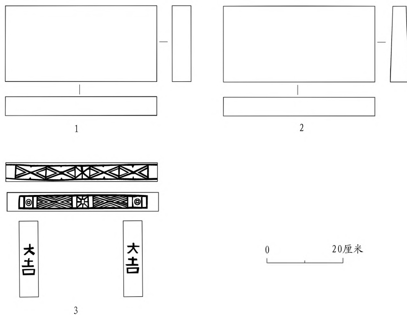
图五// M2墓砖及纹饰
