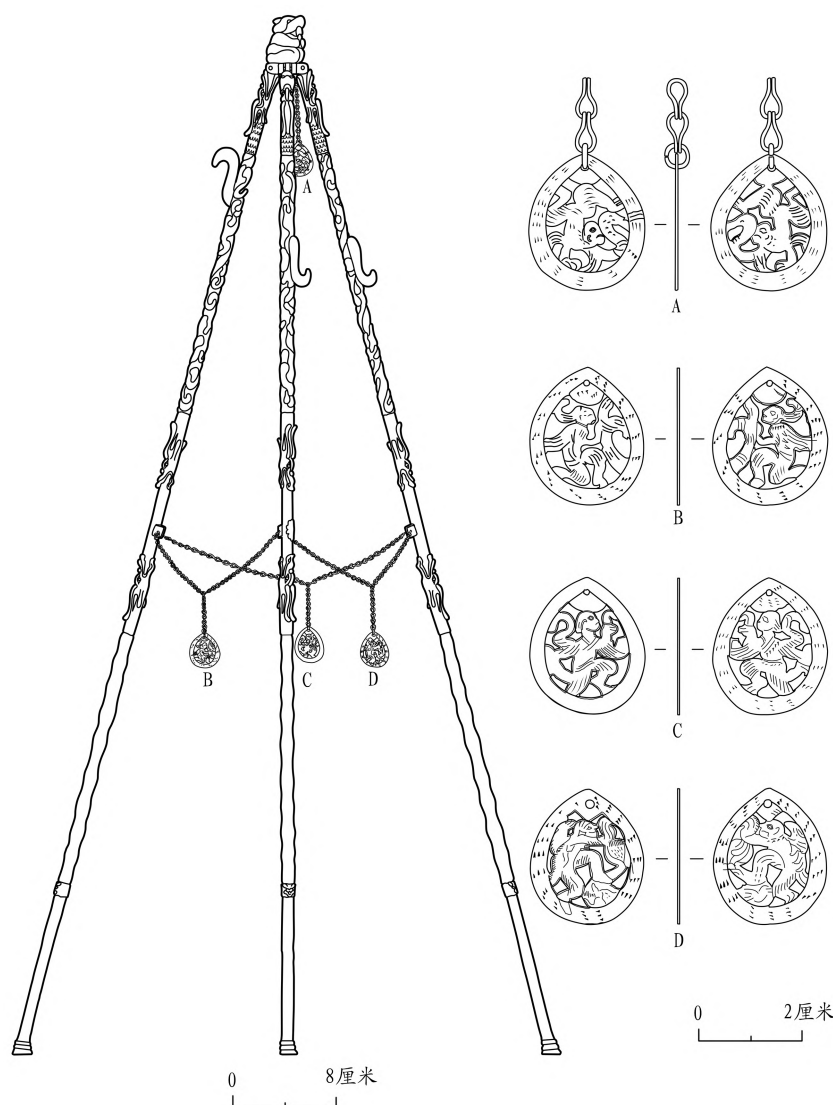
图一二// M2出土银鎏金三足镜架(M2:29)
